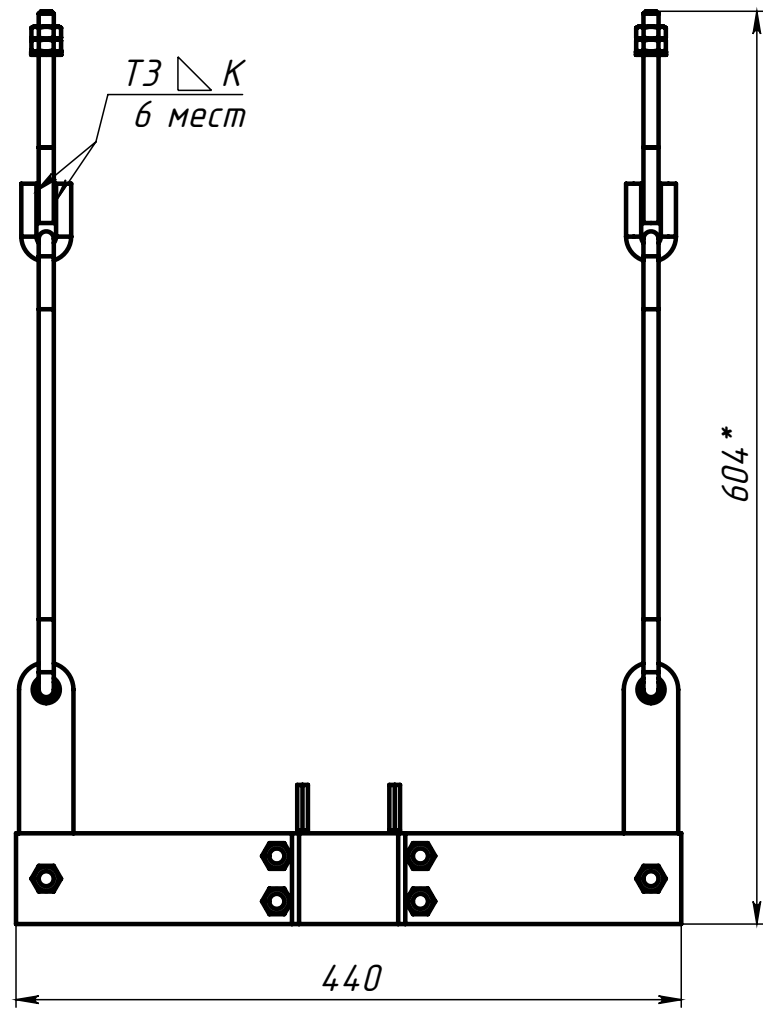
Поз.1 (Полухомут)
