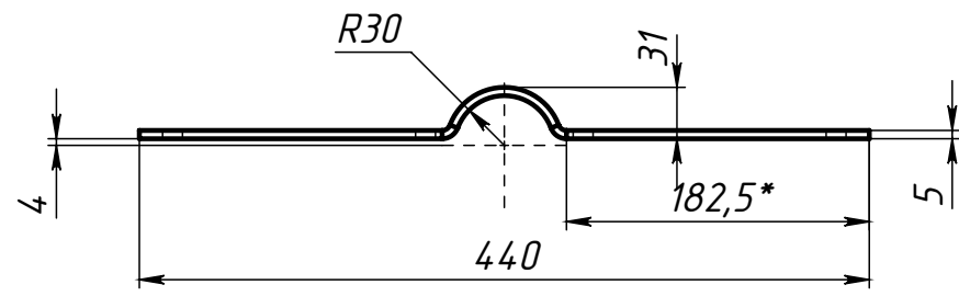
Поз.1 (Полухомут) развертка
