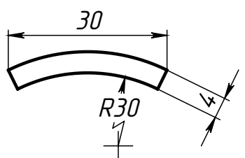
Поз.2 (Упор) 1:1
