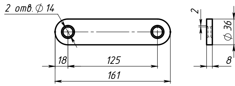
Поз.3 (Серьга) 1:3
